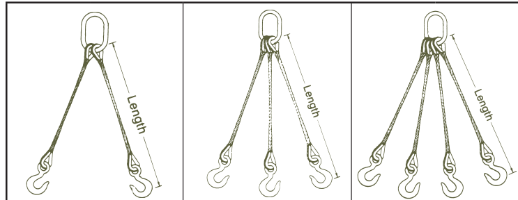
2-Leg Bridle
