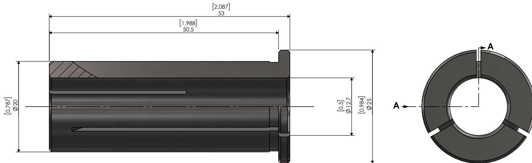
SECTION A-A
