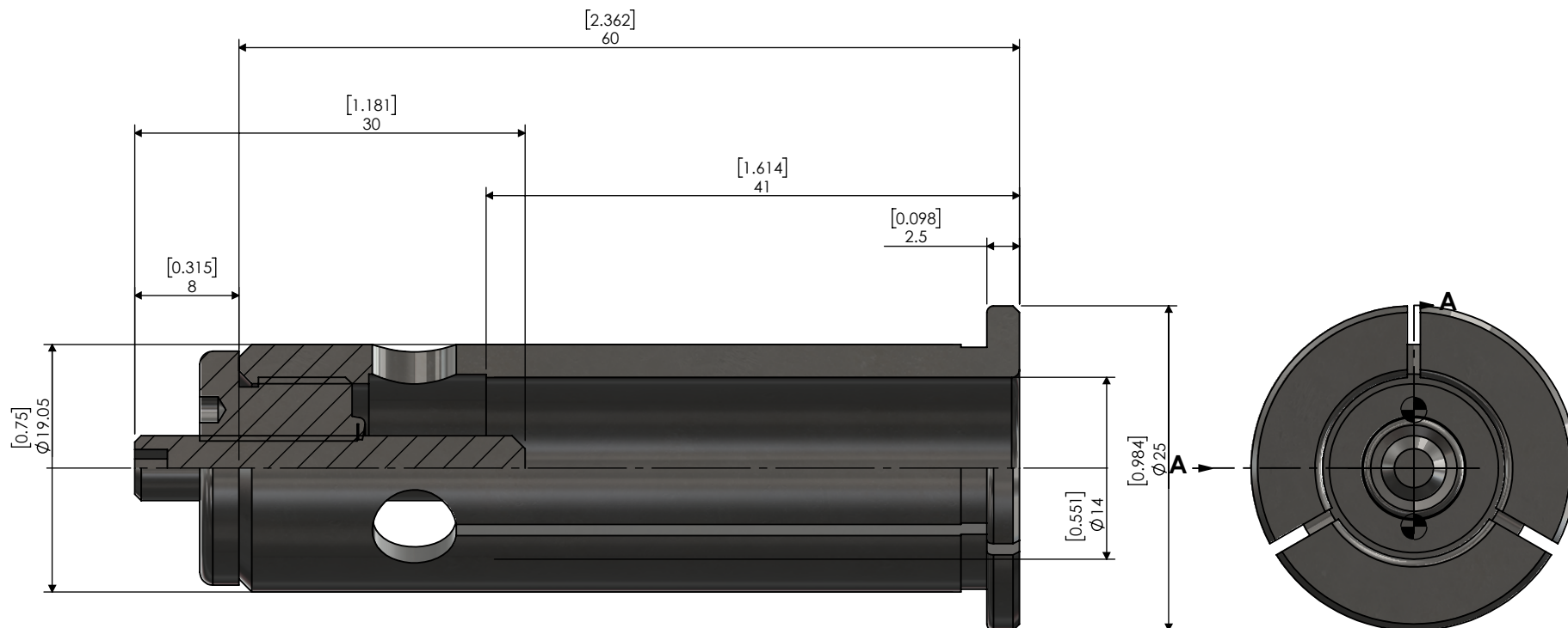
SECTION A-A
