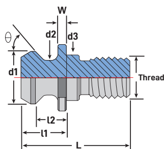
MegaFORCE ANSI/ISO Style
