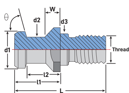
MegaFORCE DIN Style
